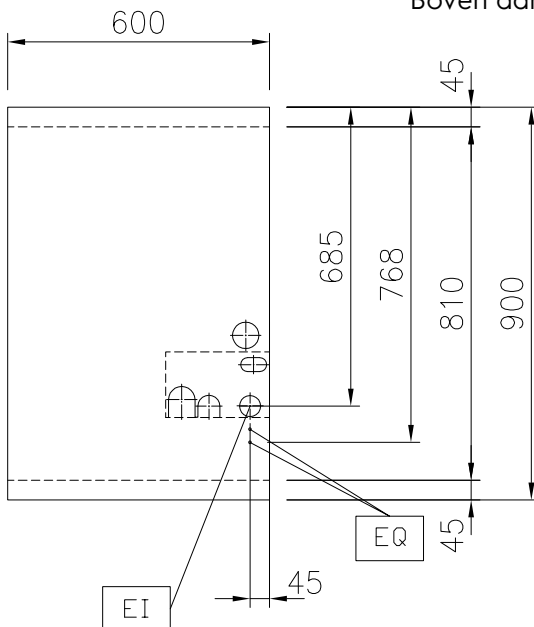
Boven aanzicht
